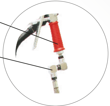
Conexão giratória Z Comando de graxa Mangueira hidráulica de 1/4 com 2 tramas de aço
